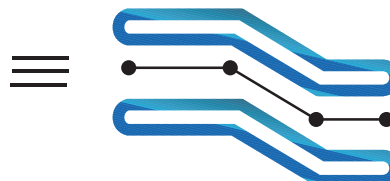
konyugatsiyalangan tizim
