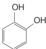
pirokateksin (benzendiol-1,2; 1,2-digidroksi- benzol)
