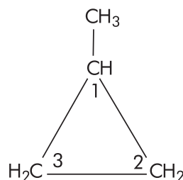
metilsiklopropan
