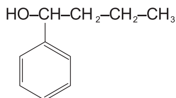
1-fenilbutanol-1
