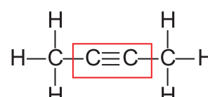
dimetilatsetilen
