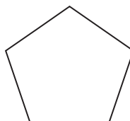
siklopentan
